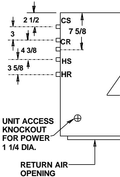
L.H. SIDE SLAVE UNIT
