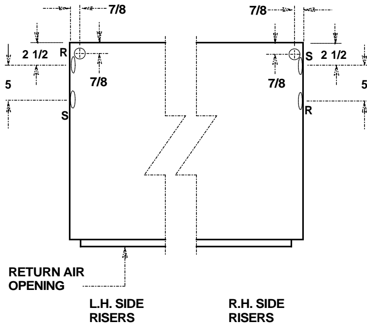
SIDE RISERS
