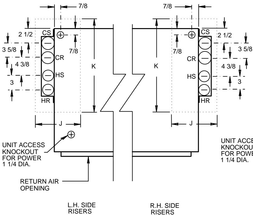
SIDE RISERS
