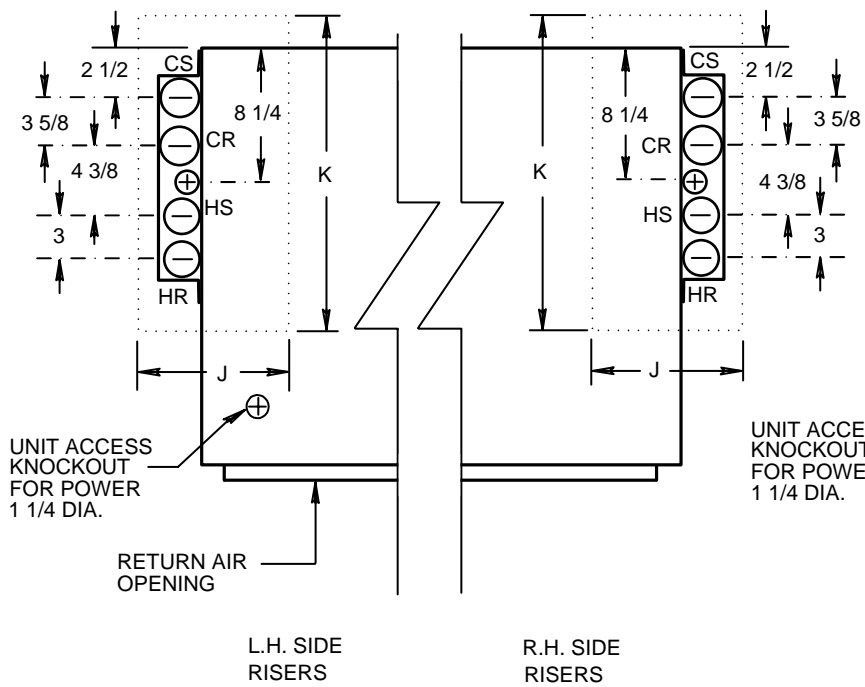
SIDE RISERS
